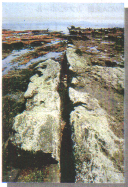
三浦活断層群 南下浦断層
