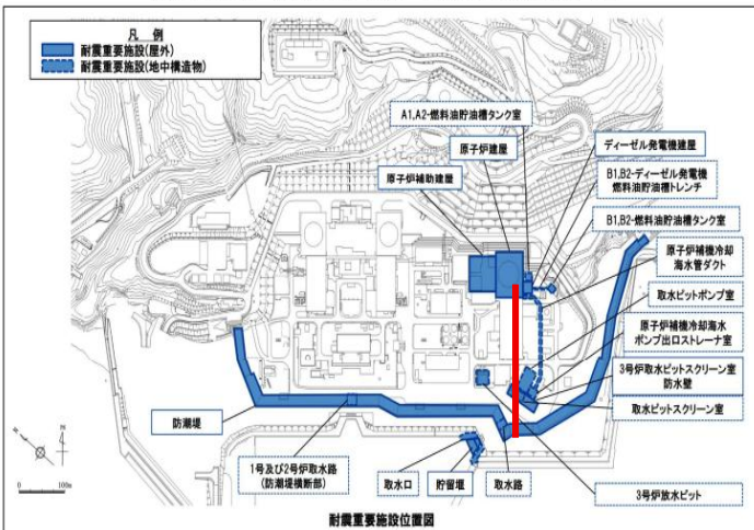
北海道電力・泊原発3号機 耐震重要施設の位置
