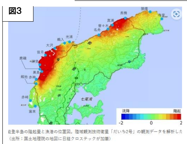
図1:音波探査では、海底活断層は図中の赤や青、黒のように切れ切れにしか認定できていなかったが、アナグリフ(図2)を用いた変動地形学的手法では、黄色の線のように、連続した1本の活断層として認定できていた。(後藤、2024; 後藤・鈴木、2024) 図3:海岸に近い海底活断層により、能登半島北岸では、最大4m以上の地震性隆起を生じた。隆起量は活断層からの距離や地盤の影響で異なるが、ほぼ1m~2mの隆起が生じている。
