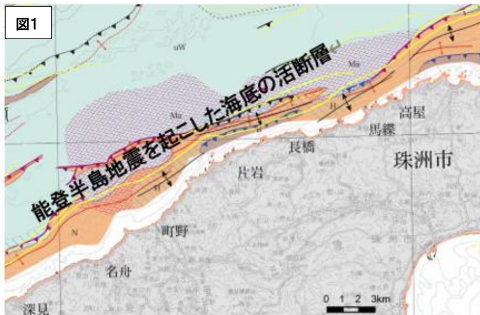
図1:音波探査では、海底活断層は図中の赤や青、黒のように切れ切れにしか認定できていなかったが、アナグリフ(図2)を用いた変動地形学的手法では、黄色の線のように、連続した1本の活断層として認定できていた。(後藤、2024; 後藤・鈴木、2024) 図3:海岸に近い海底活断層により、能登半島北岸では、最大4m以上の地震性隆起を生じた。隆起量は活断層からの距離や地盤の影響で異なるが、ほぼ1m~2mの隆起が生じている。
