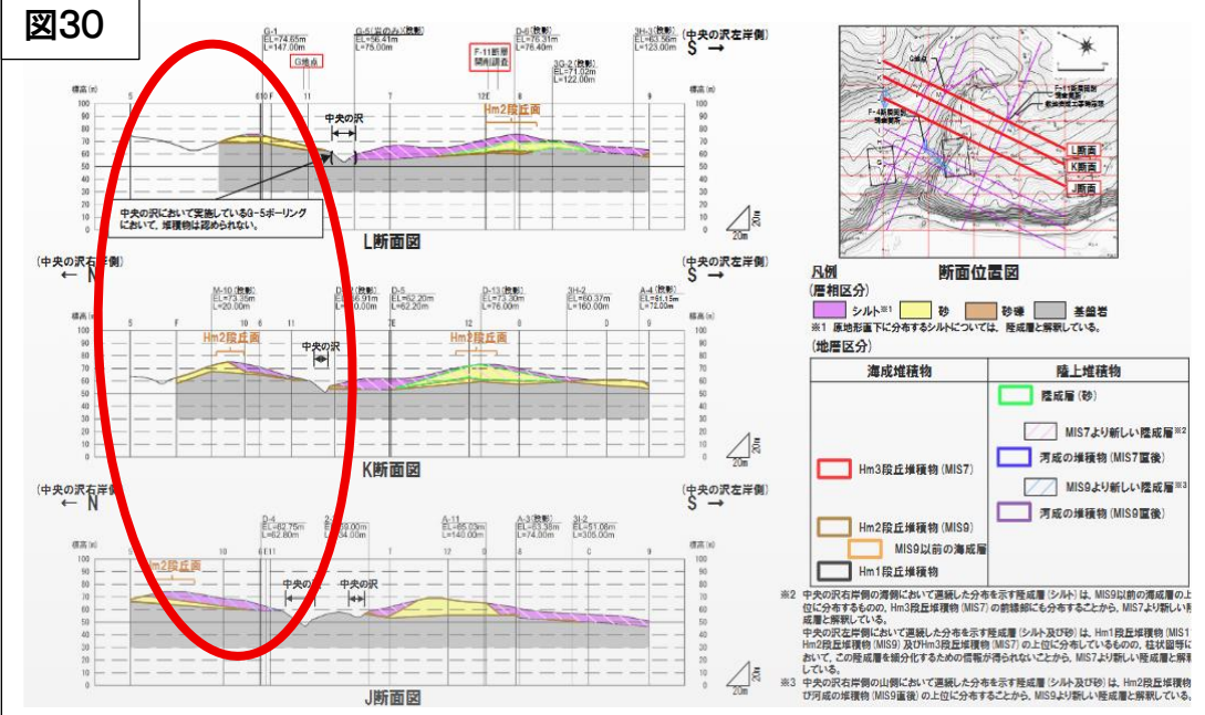
③-1 中央の沢付近のHm2段丘堆積物の分布状況 -断面図 (2/4) -
